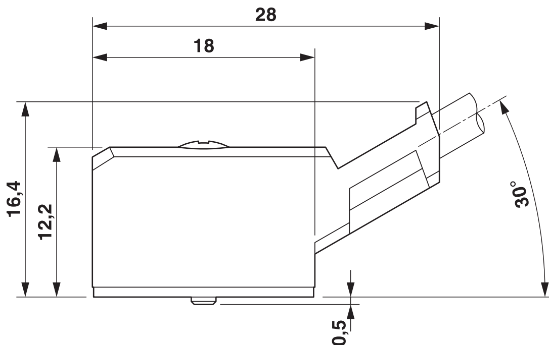
Rysunek wymiarowy
