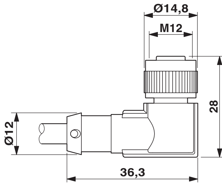
Rysunek wymiarowy
