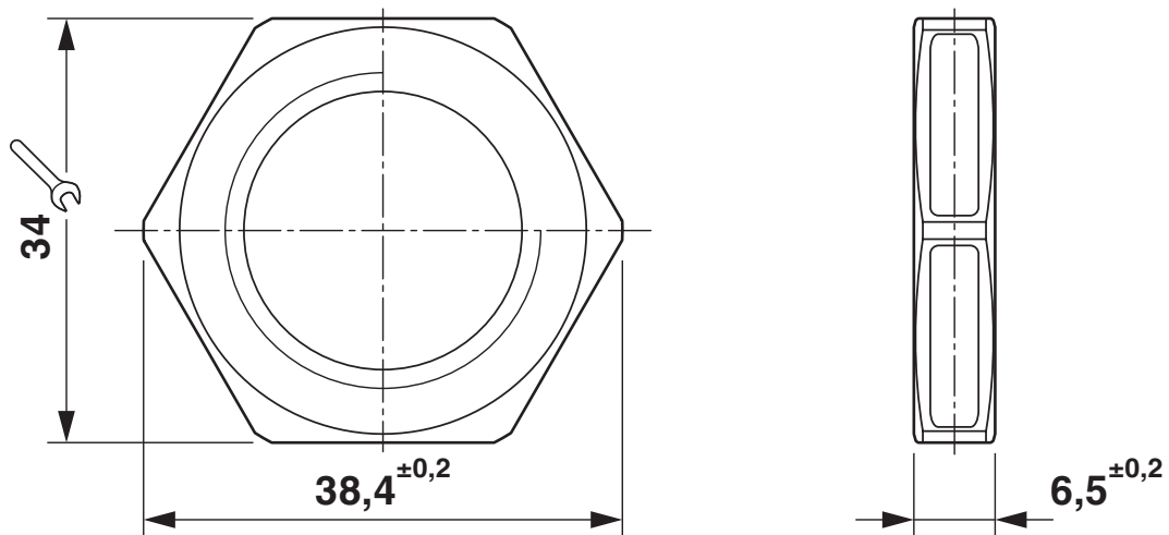
Rysunek wymiarowy
