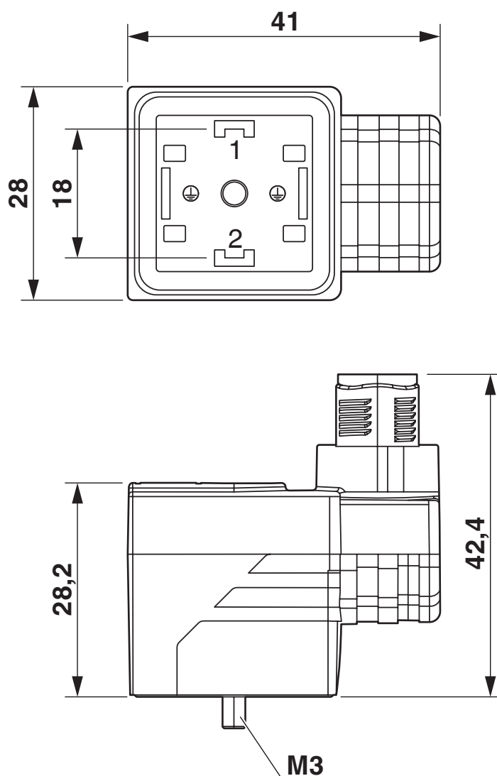
Rysunek wymiarowy
