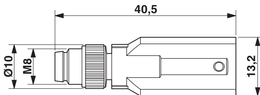
Rysunek wymiarowy
