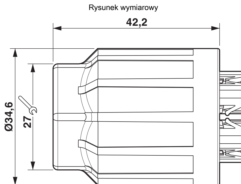
Rysunek wymiarowy nakrętki QPD 5x2,5
