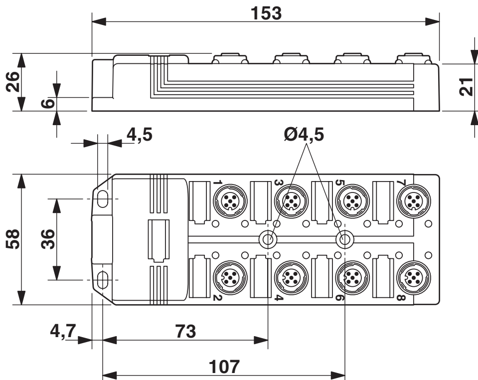
Rysunek wymiarowy
