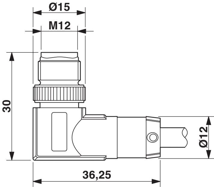
Rysunek wymiarowy
