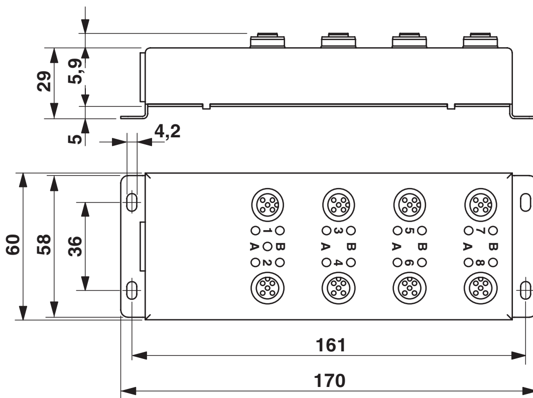
Rysunek wymiarowy
