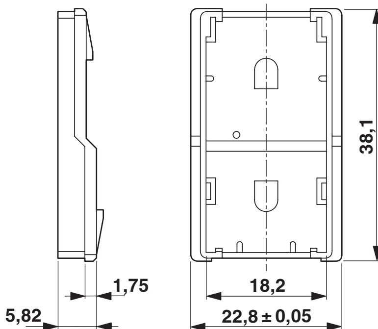
Rysunek wymiarowy
