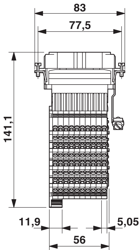
Rysunek wymiarowy
