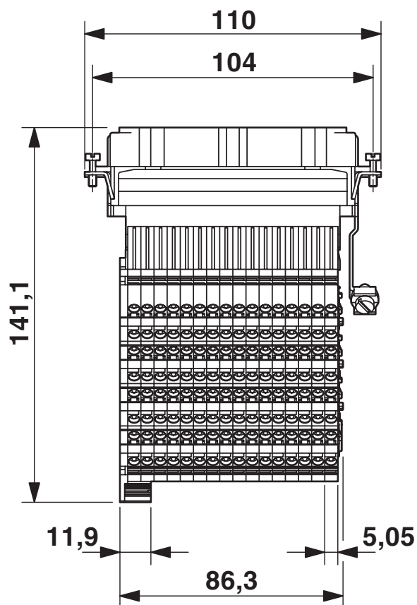
Rysunek wymiarowy
