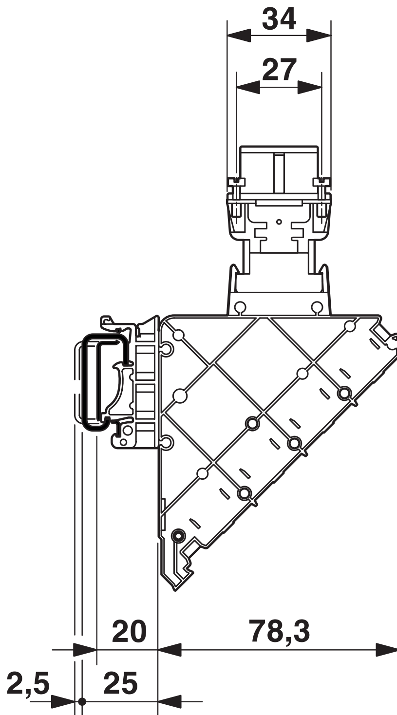
Rysunek wymiarowy
