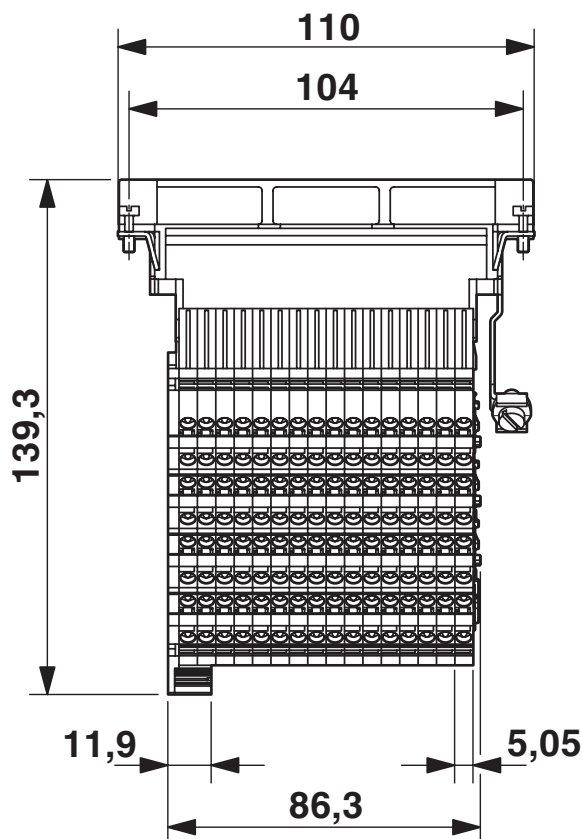
Rysunek wymiarowy
