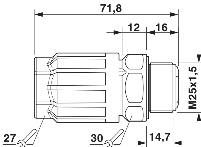
Rysunek wymiarowy
