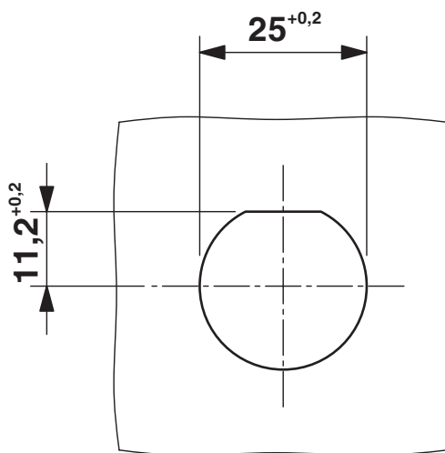
Rysunek wymiarowy
