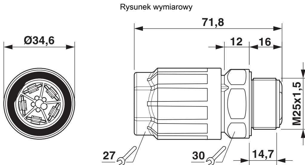
Rysunek wymiarowy QPD W 4PE2,5 M25
