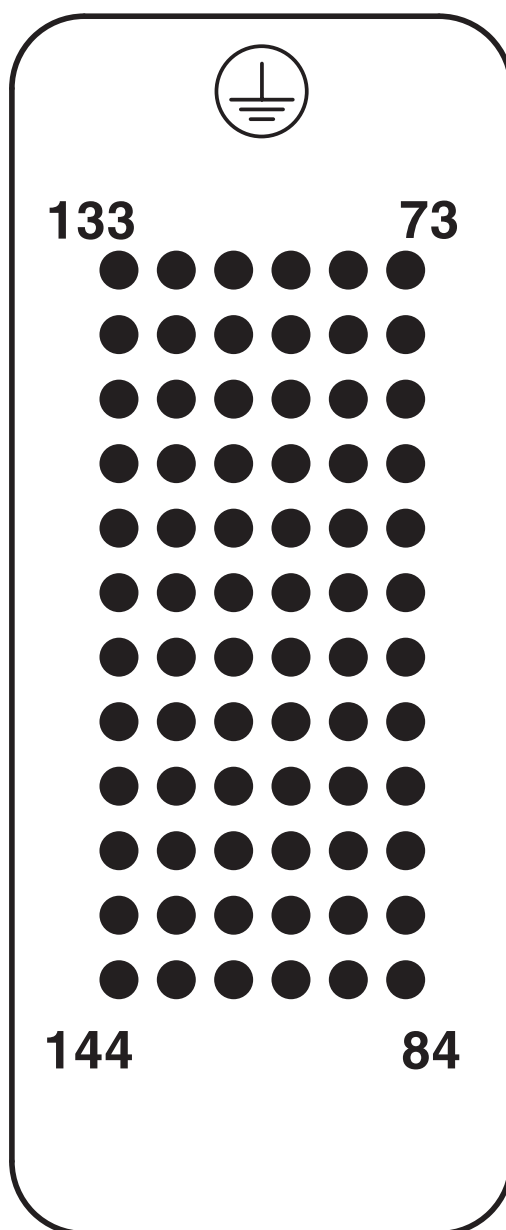
Rysunek schematyczny
