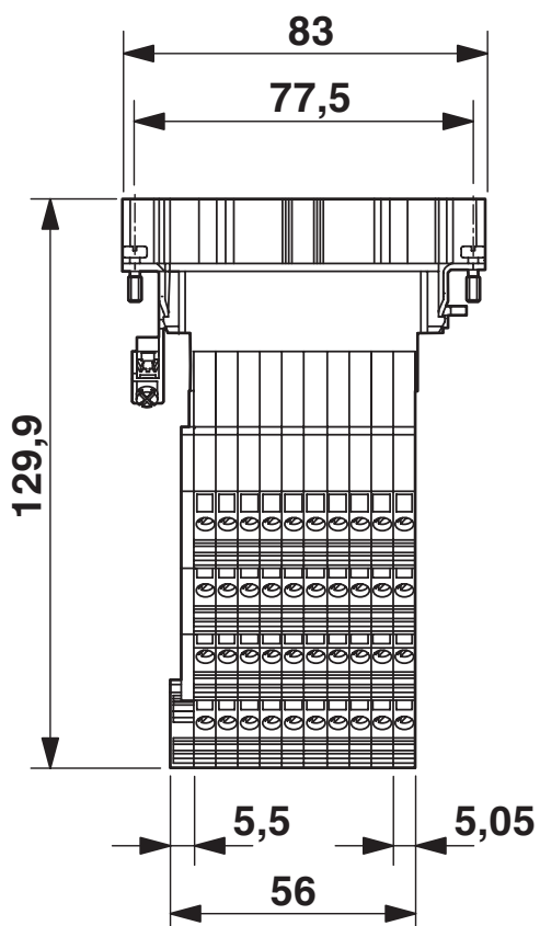
Rysunek wymiarowy
