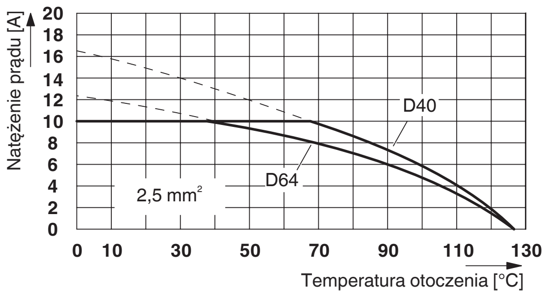
Krzywa redukcyjna dla 2,5mm 2
