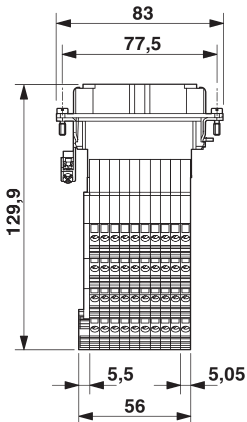
Rysunek wymiarowy
