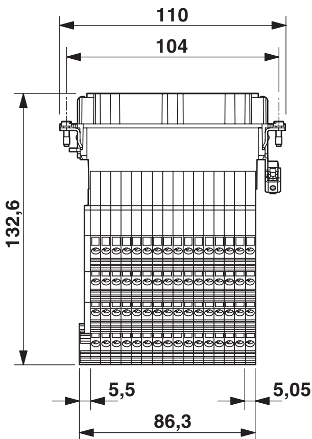
Rysunek wymiarowy
