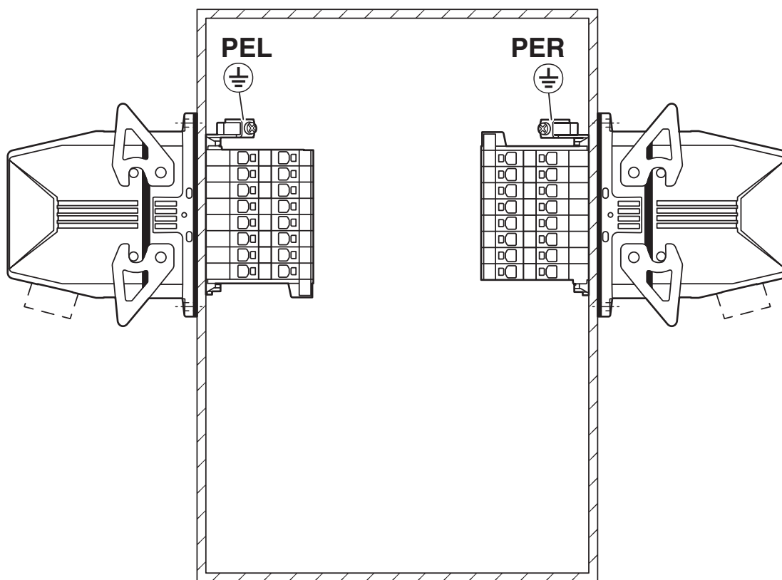
rysunek aplikacji
