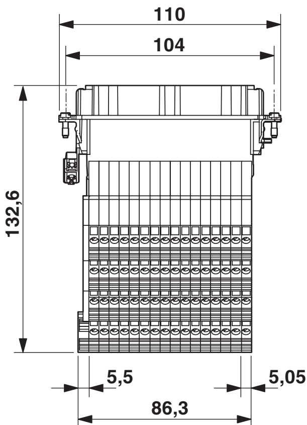
Rysunek wymiarowy
