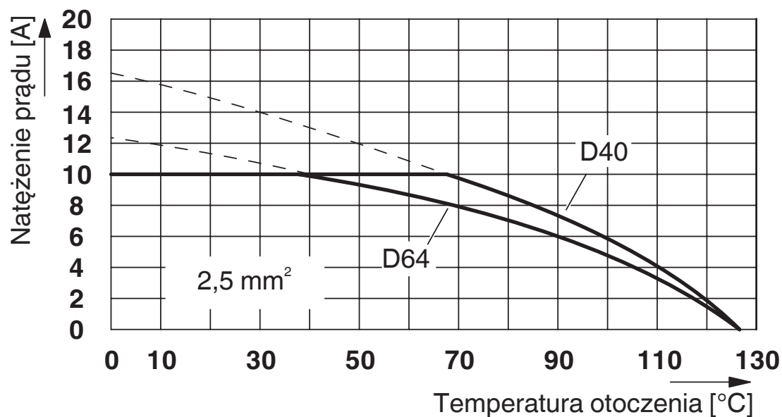
Krzywa redukcyjna dla 2,5mm²
