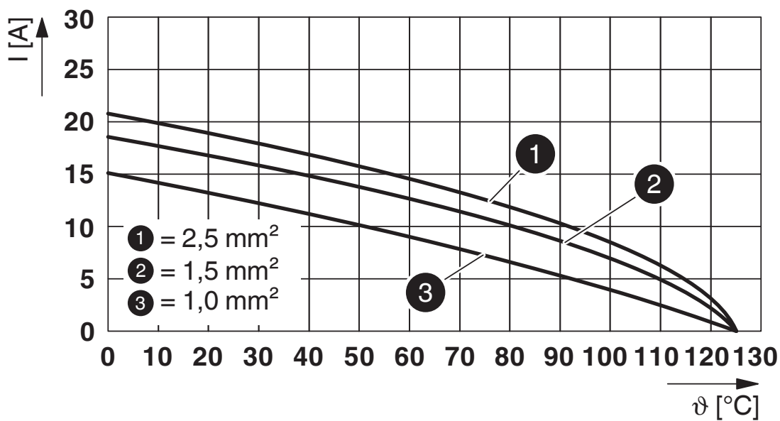
Wykres obniżenia parametrów znamionowych styków zwijanych
