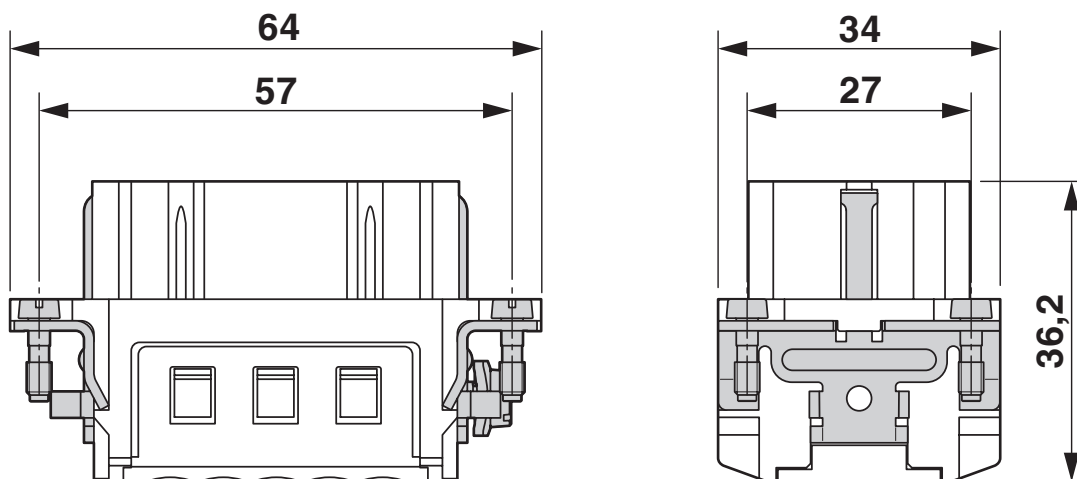
Rysunek wymiarowy
