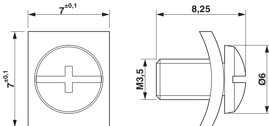
Rysunek wymiarowy
