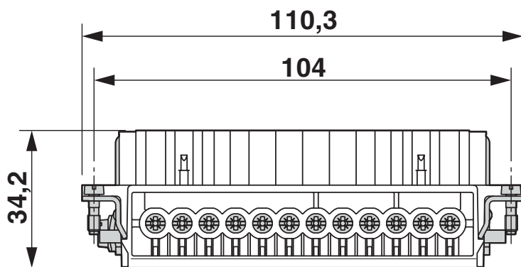
Rysunek wymiarowy
