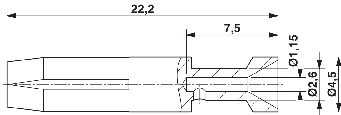
Rysunek wymiarowy
