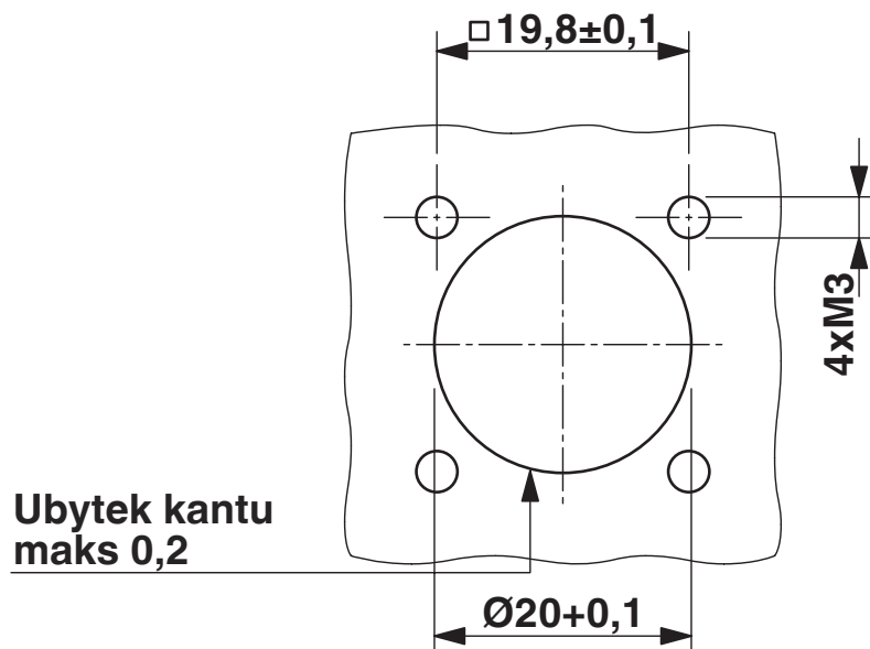
Rysunek wymiarowy
