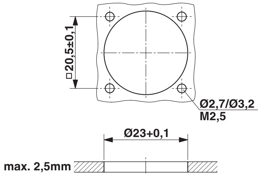
Rysunek wymiarowy
