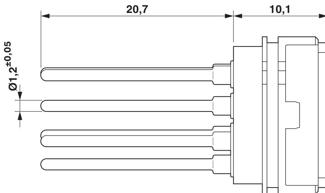
Rysunek wymiarowy
