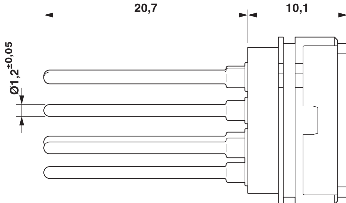
Rysunek schematyczny
