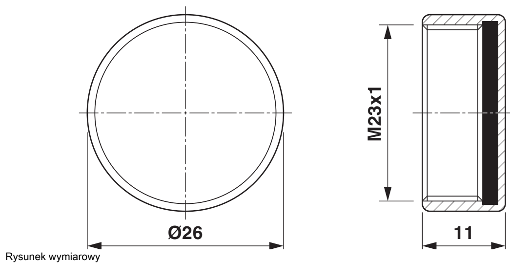
Rysunek wymiarowy
