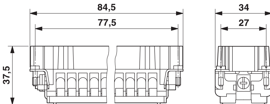
Rysunek wymiarowy
