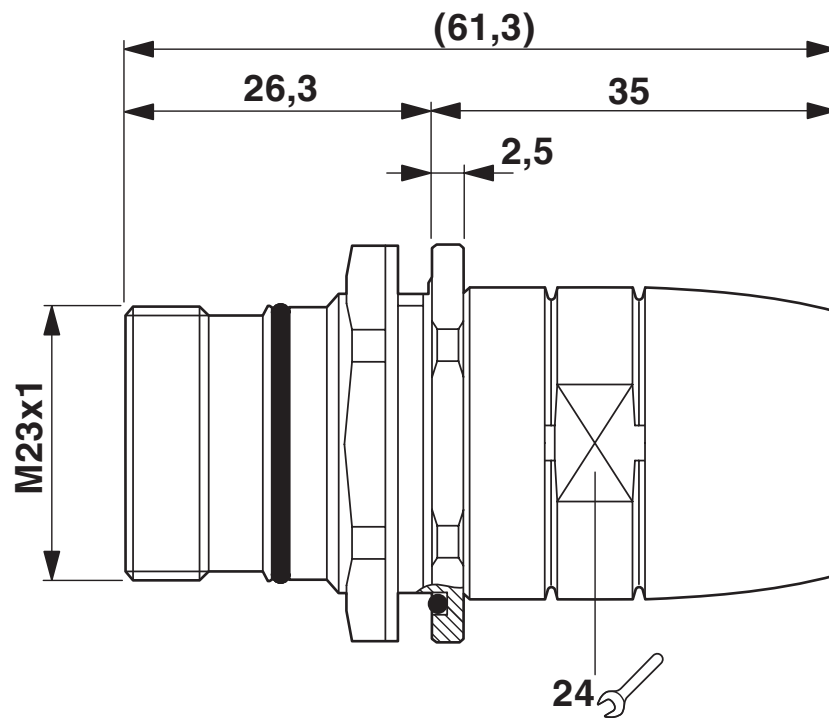
Rysunek wymiarowy
