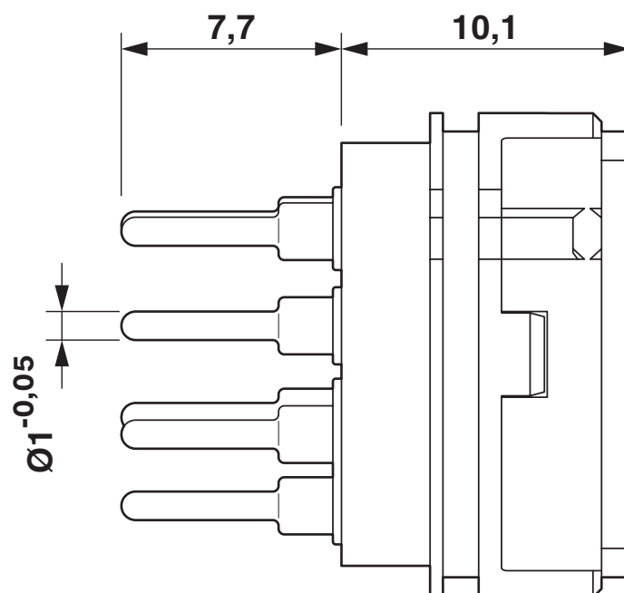
Rysunek wymiarowy
