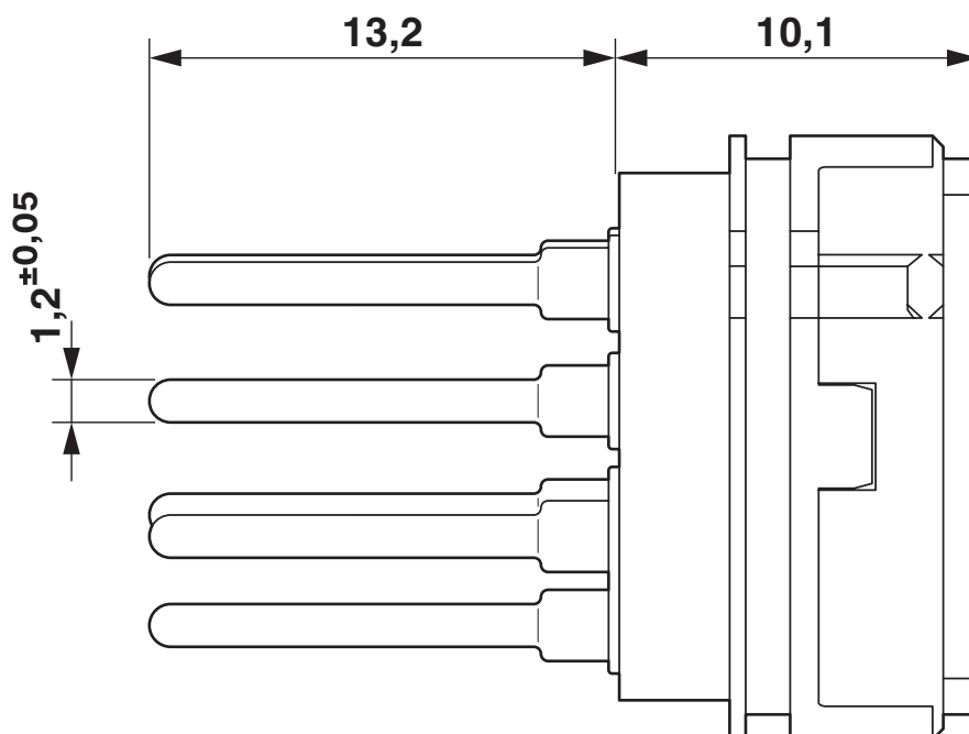
Rysunek wymiarowy
