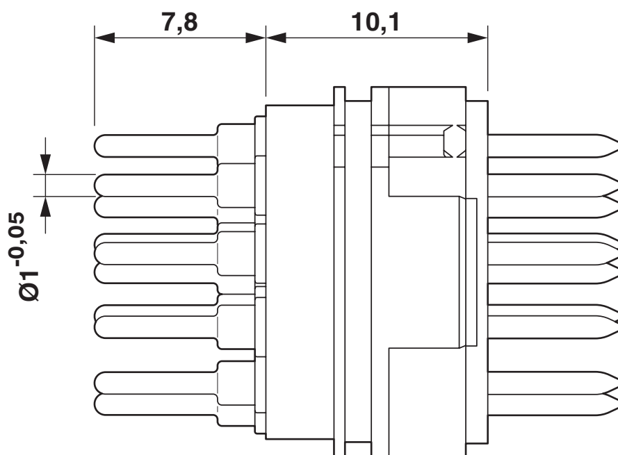
Rysunek wymiarowy
