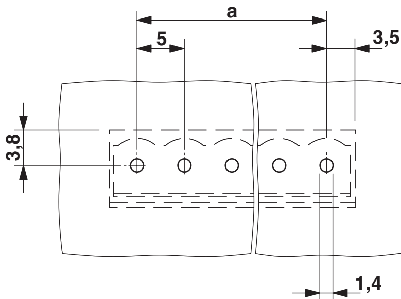
Otworowanie/geometria płytek lutowiczych
