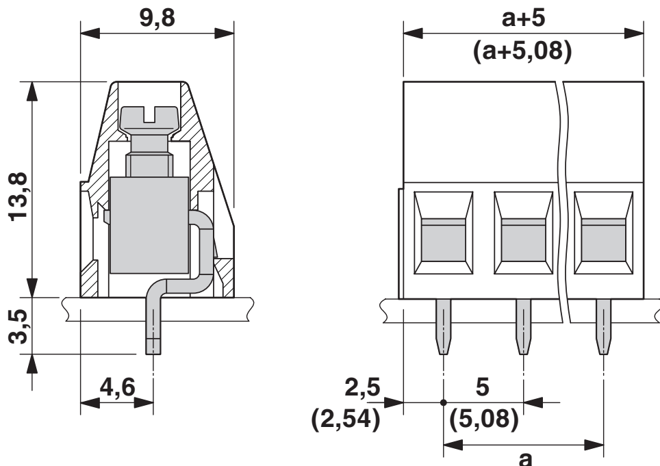
Rysunek wymiarowy
