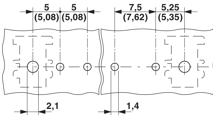
Otworowanie/geometria płytek lutowniczych
