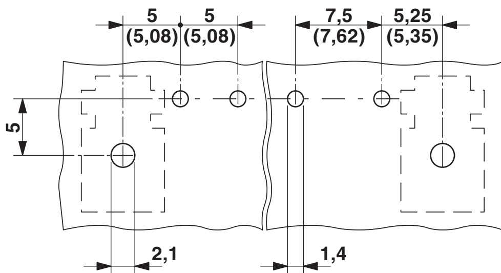
Otworowanie/geometria płytek lutowniczych
