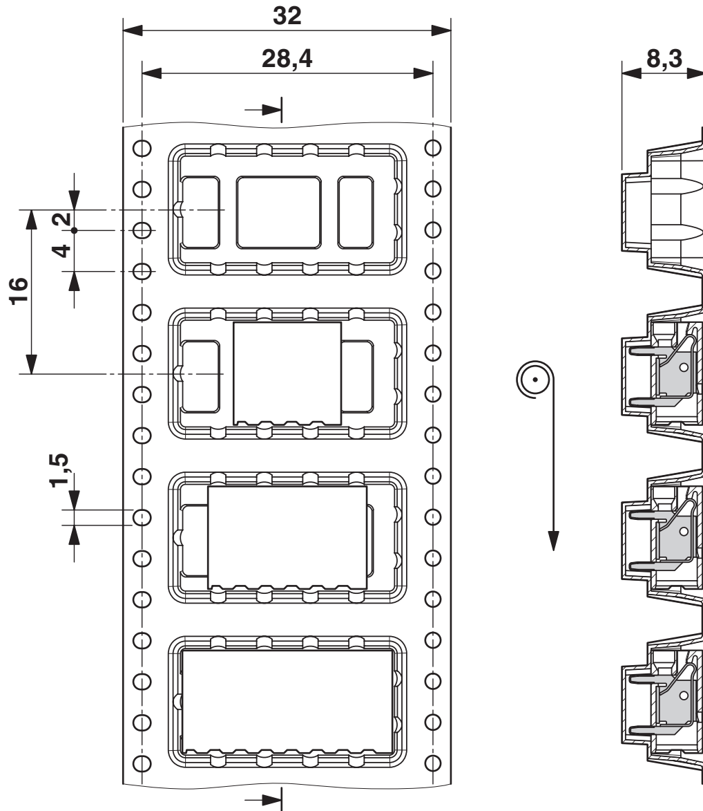
Rysunek wymiarowy
