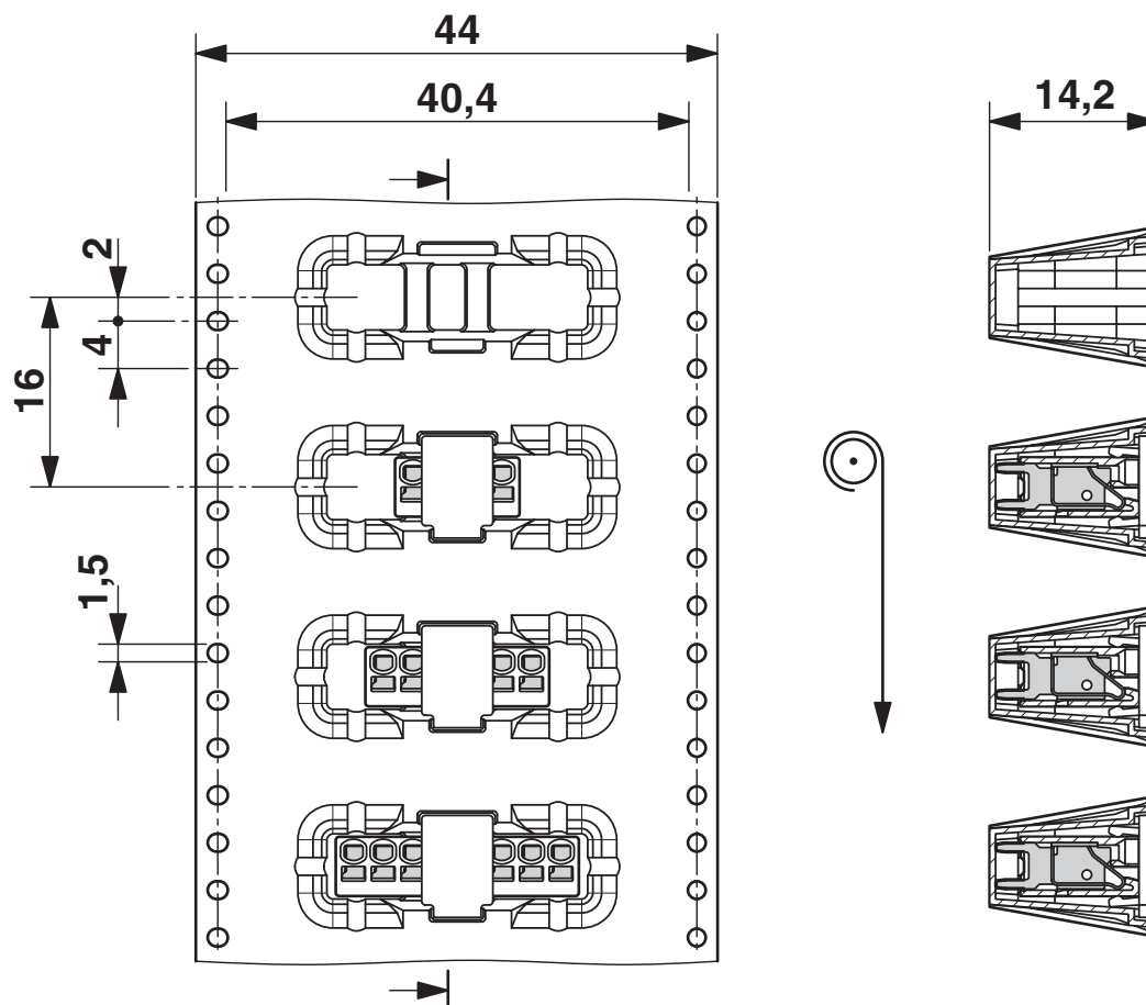
Rysunek wymiarowy
