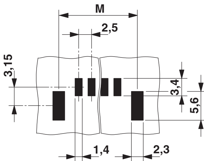
Otworowanie/geometria płytek lutowniczych
