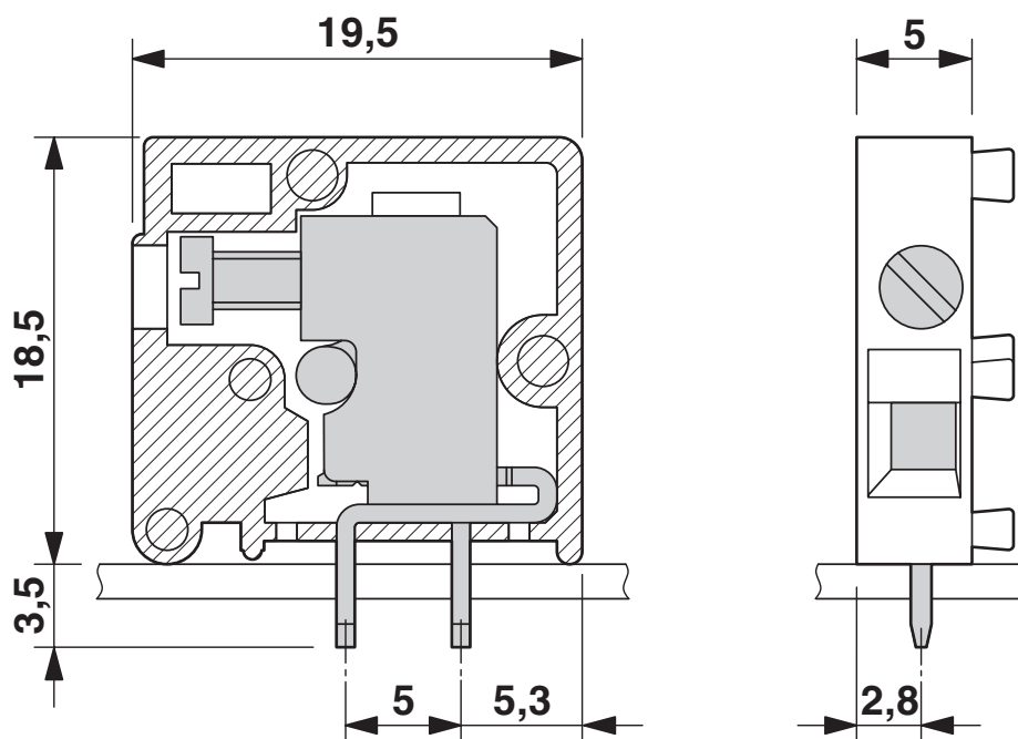
Rysunek wymiarowy
