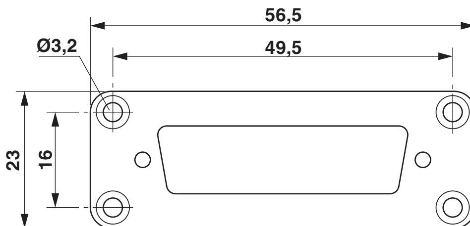
Rysunek wymiarowy
