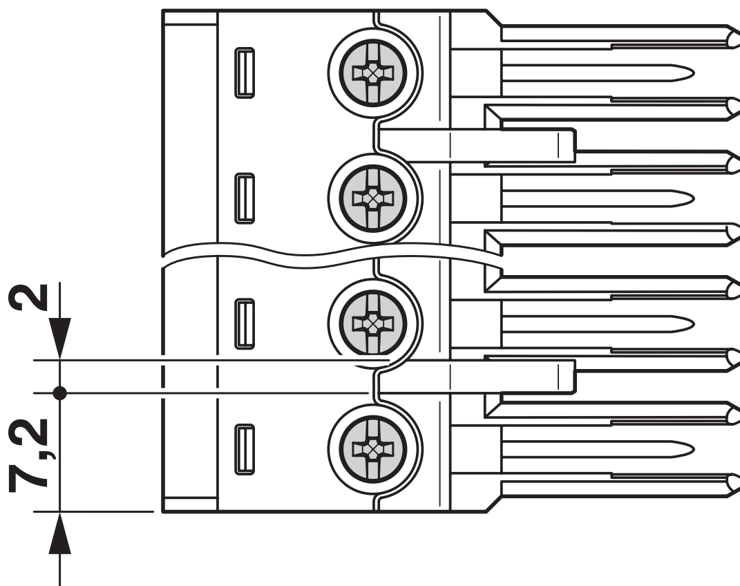
Rysunek wymiarowy
