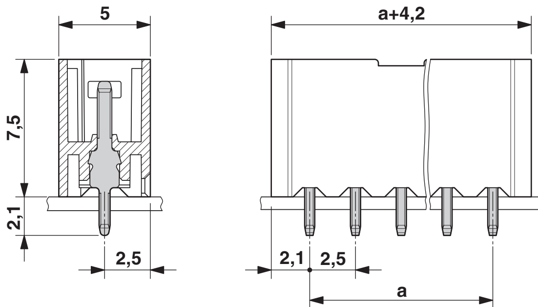
Rysunek wymiarowy
