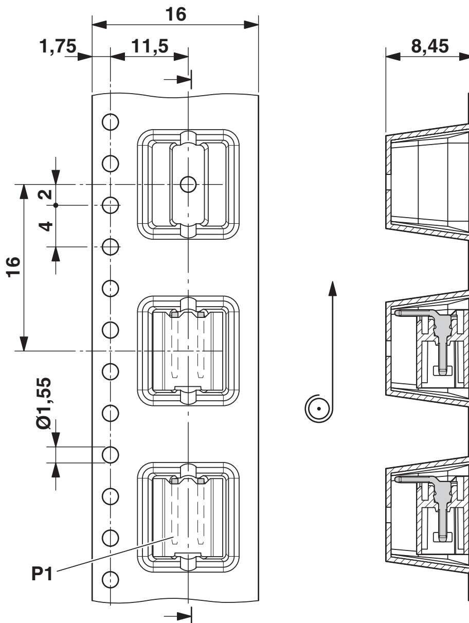
Rysunek wymiarowy
