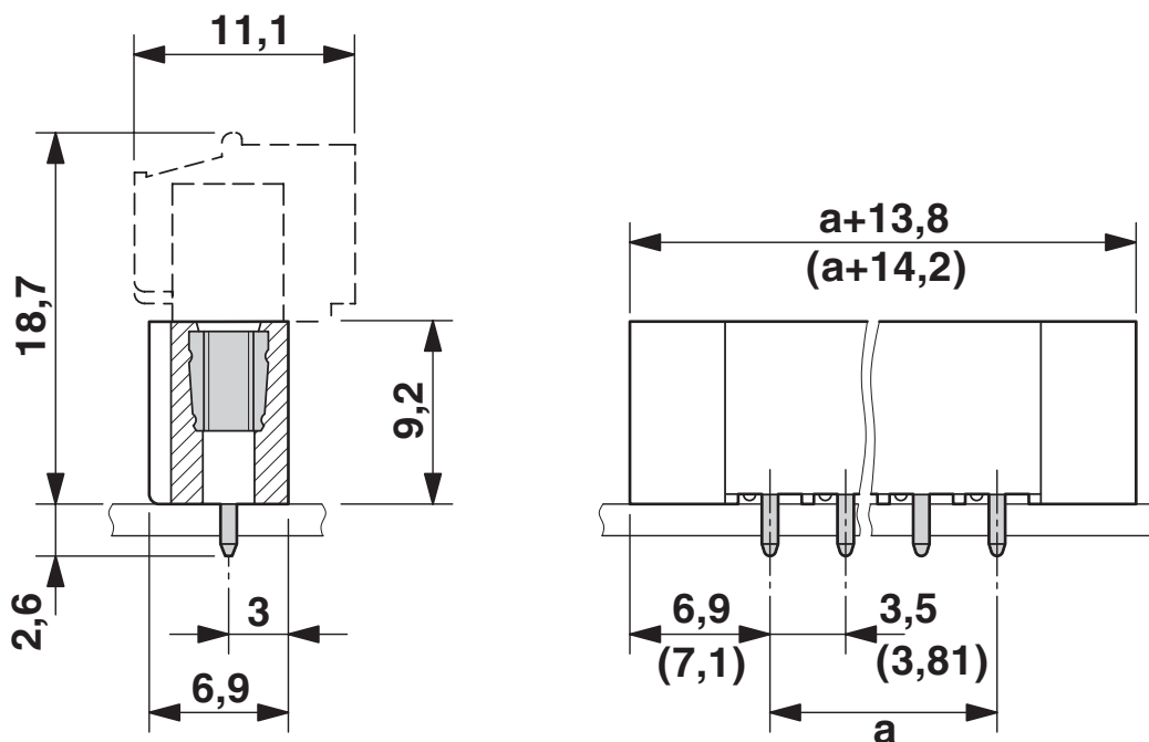
Rysunek wymiarowy
