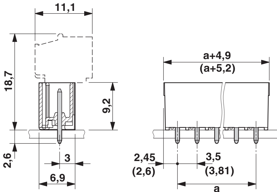
Rysunek wymiarowy
