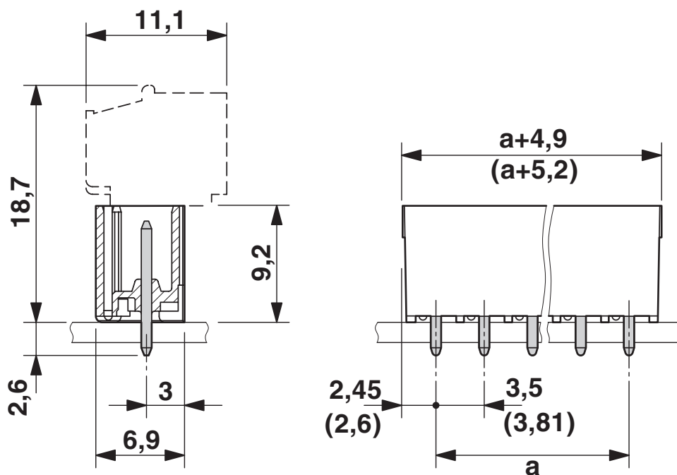
Rysunek wymiarowy
