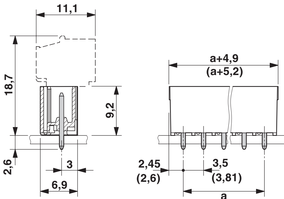
Rysunek wymiarowy
